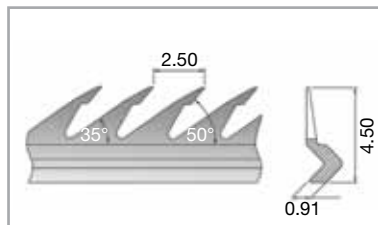
VF28/250/50 SiroLock®
